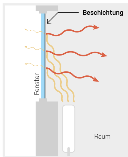
Heizwärme-Gewinn durch Reflexion in den Raum.
